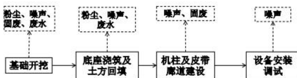
图 3.2-1 皮带廊施工工艺流程及产污环节图
