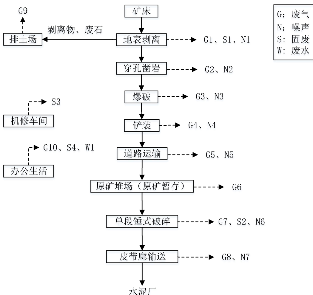
图 3.1-1 项目生产工艺及产污环节图
