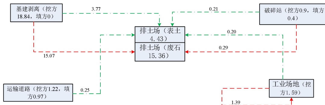
图 3.2-2 施工期土石方平衡图 单位：万 m 3
