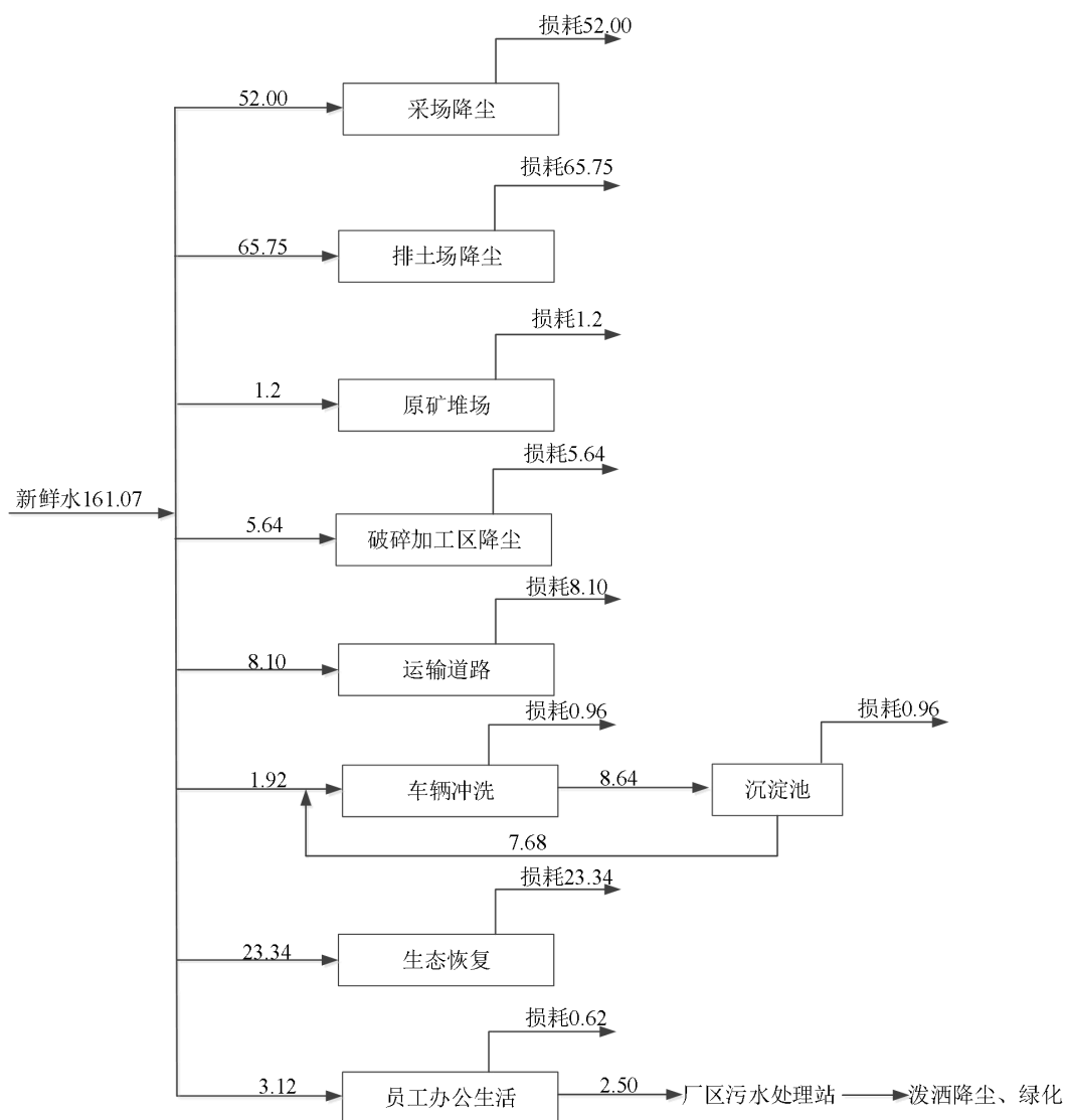
图 2.6-1 项目水平衡图 单位：m³/d
