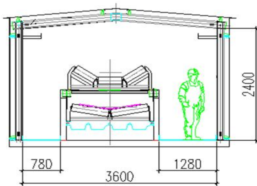
图 2.4-2 皮带廊道横断面图 单位：mm
