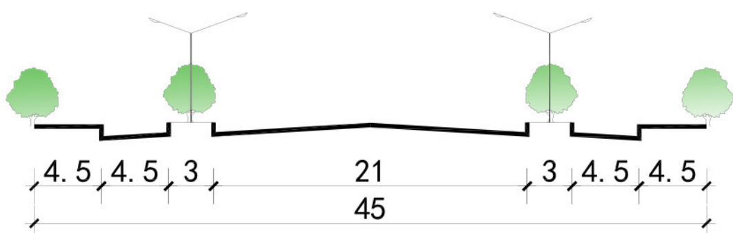
A-A(南二环路) 道路横断面
