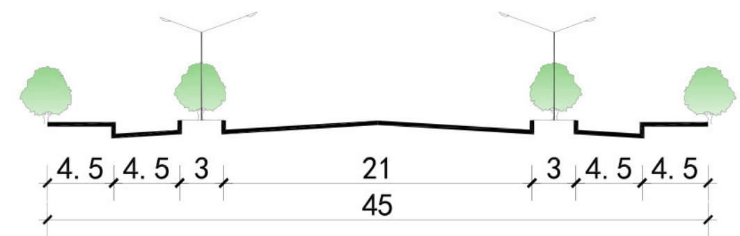
B-B(西环路、祁连路) 道路横断面
