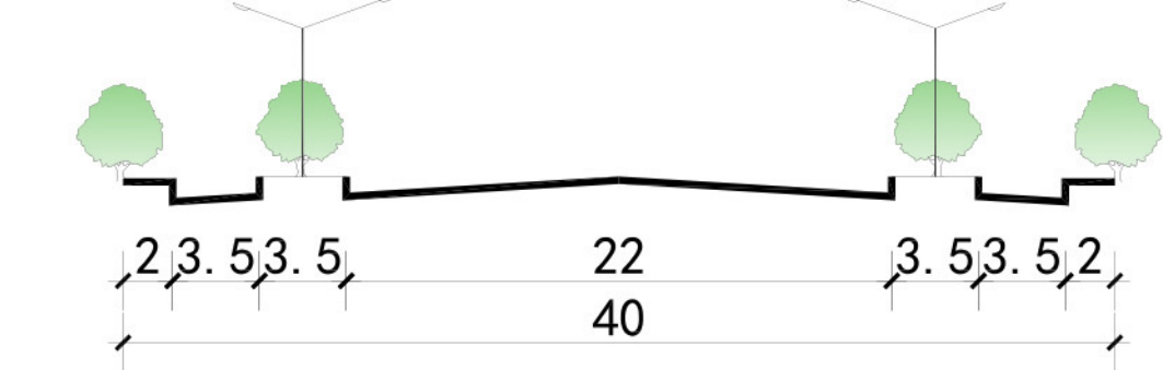
D-D(西域西路西段) 道路横断面
