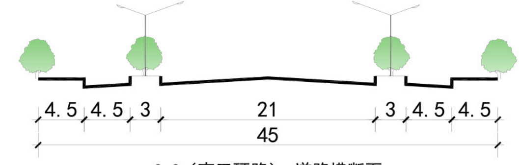
C-C(南三环路) 道路横断面
